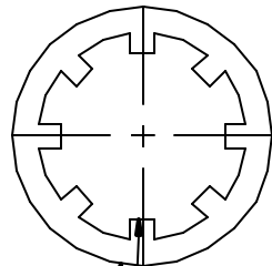
7.80 [ø.307] 5.00 [ø.197]
