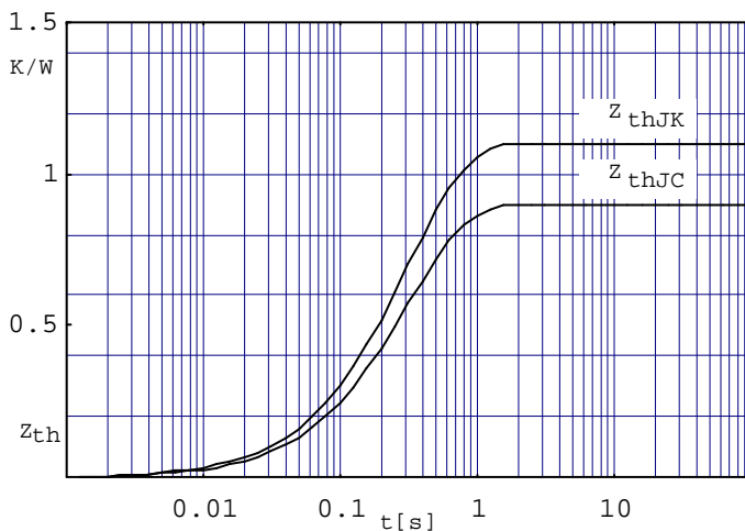
Fig. 6 Transient thermal impedance per diode
