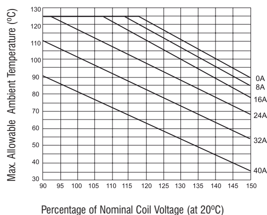
MAX. ALLOWABLE AMBIENT TEMPERATURE (°C)
