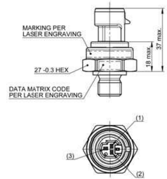
Packard (Metri-Pack 150)
