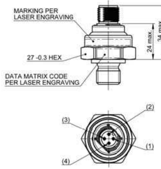
M12 - 4 Pole
