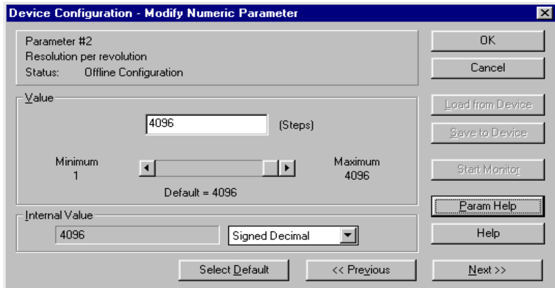
Figure 5 Parameter mask
