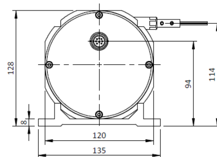
C connection (Connector M16 - DIN 8 pin)
