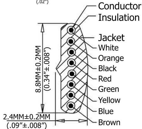
SEC: A-A
