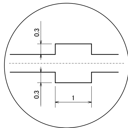
ストッパー部詳細図 Detail of stopper
