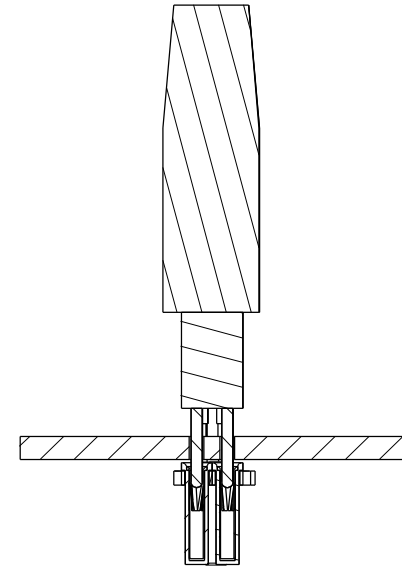
Section D-D
