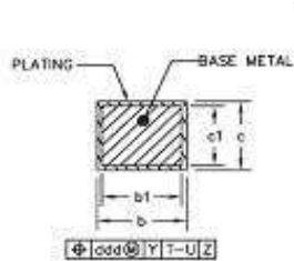
SECTION G-G SCALE: 100/1
