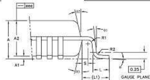
DETAIL F SCALE: 20/1
