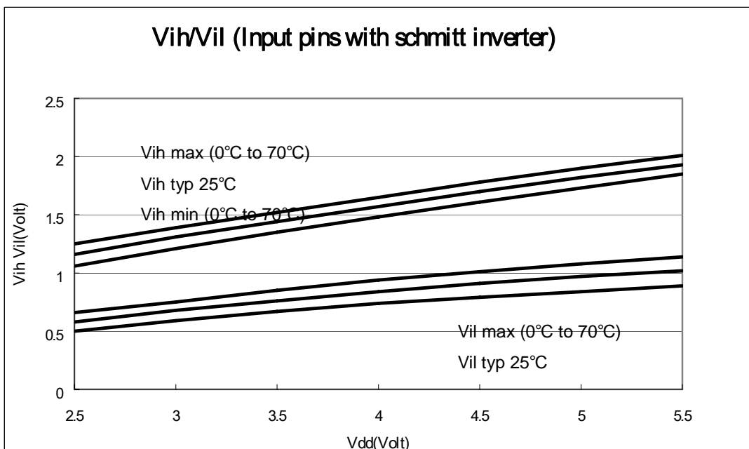
Fig. 17 Vih, Vil of Port6 vs. VDD
