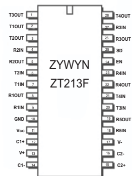
28-pin SSOP/WSOIC
