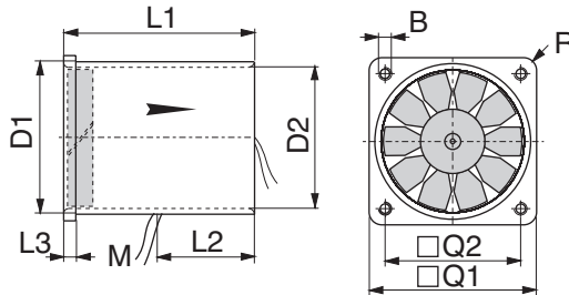
D301Q, D303Q, D304Q 12 VDC
