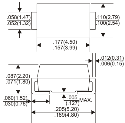
DO-214AC(SMA)
