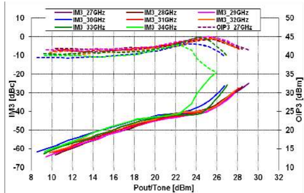
@ V_{ds}=4V , I_{dsq}=3.1A
