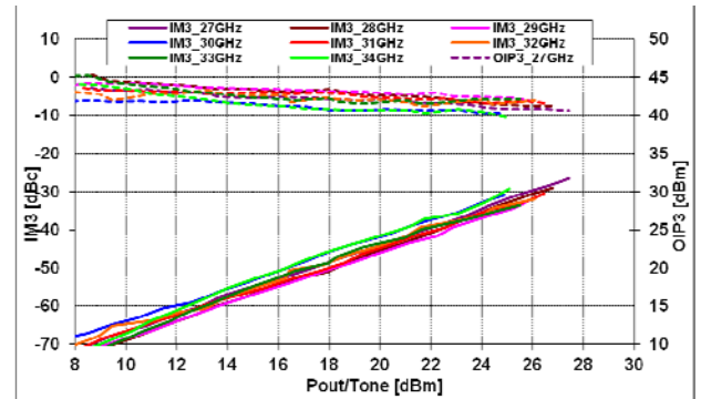
@ V_{ds}=4V , I_{dsq}=2.2A
