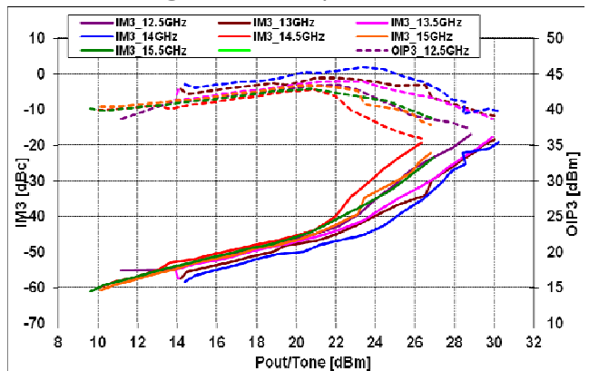
@ V_{ds}=5V , I_{dsq}=2500mA
