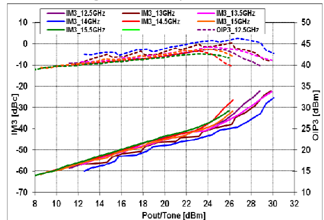
@ V_{ds}=6V , I_{ds}=2500mA
