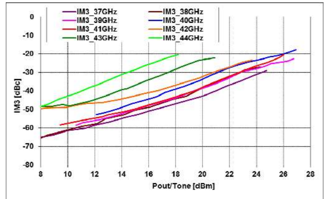
IM3 Level(dBc) vs. Pout/tone(dBm) (Vds=5V, Idsq=1.1A)
