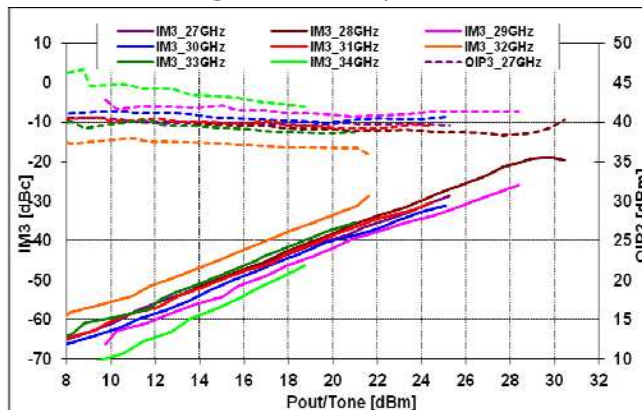
@ V_{ds}=6V , I_{dsq}=2A
