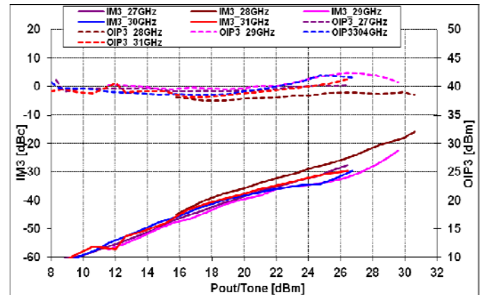
@ V_{ds}=5V , I_{dsq}=1.5A
