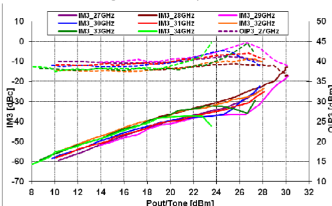
@ V_{ds}=4V , I_{dsq}=2.2A
