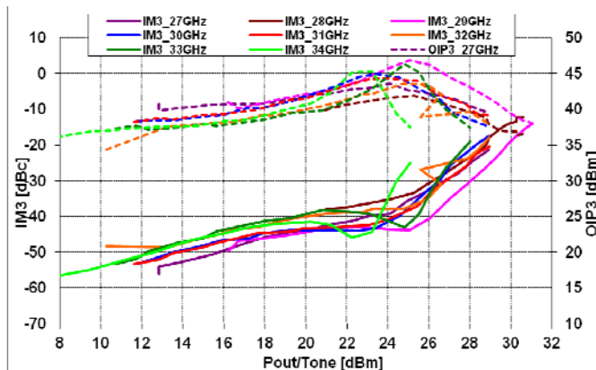
@ V_{ds}=4V , I_{dsq}=2.8A
