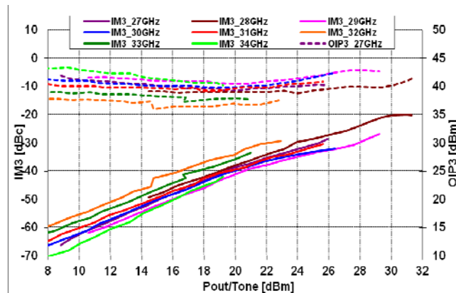
@ V_{ds}=6V , I_{dsq}=2.5A
