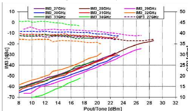
@ V_{ds}=6V , I_{dsq}=1.5A
