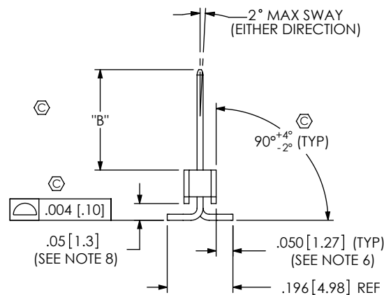
FIG 1 FTR-1XX-XX-X-S SHOWN
