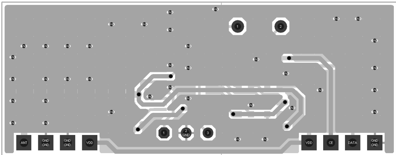
<Bottom Side>
