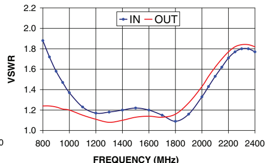
ZX60-2411BM+ VSWR
