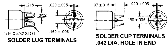
OPTIONAL TERMINAL STYLES
