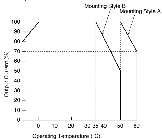
PS5R-F/G
