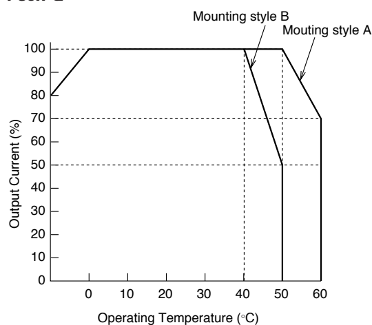
PS5R-Q
