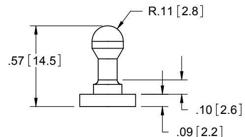
P/N: CS-113-5 STRIKER 1. MATERIAL: NYLON 6/6 (RMS-01). 2. COLOR: NATURAL.
