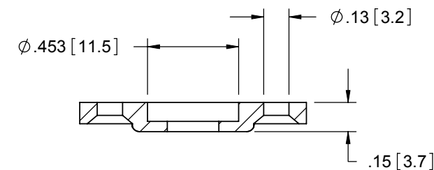
P/N: CS-113-3 BASE 1. MATERIAL: ACETAL (RMS-39). 2. COLOR: BLACK.
