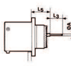
Receptacle type 3
