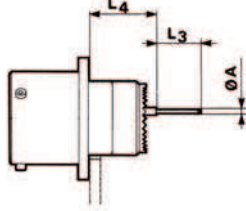
Receptacle type 0
