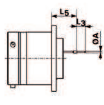
Receptacle type 2
