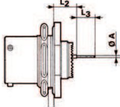
Receptacle type 7
