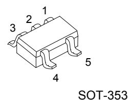
SOT-25
