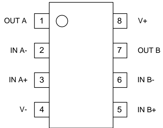
SOP-8 / TSSOP-8 / MSOP-8
