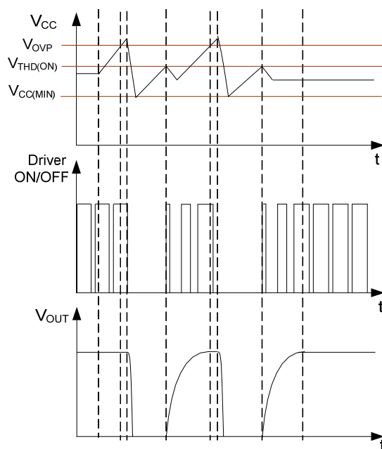
FIG.7 OVP case
