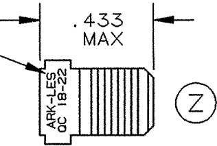
VIEW A-A
