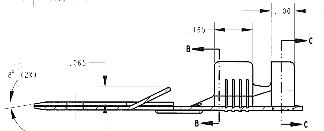
SECTION D-D
