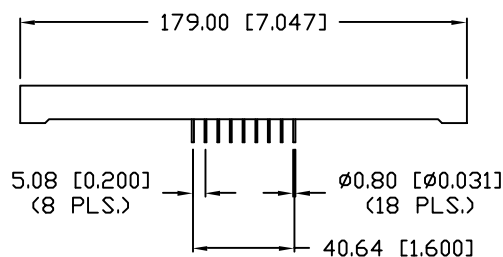
DIGIT DETAIL
