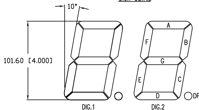
DIGIT DETAIL
