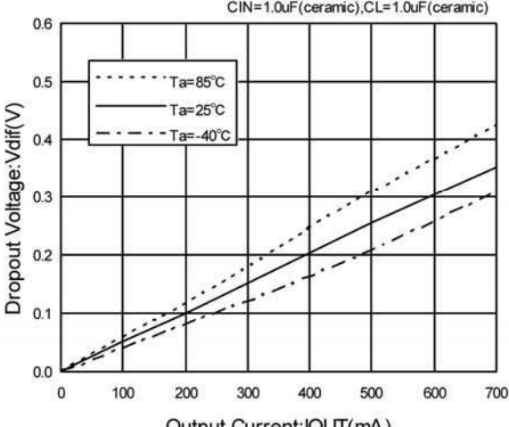
XC6210 (VOUT:3.0V)
