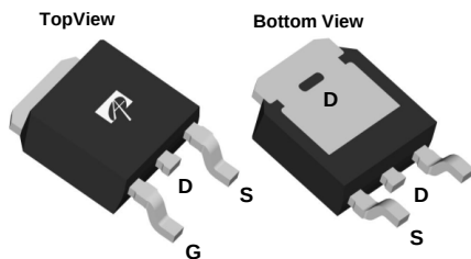
TO252 DPAK: AOD516
