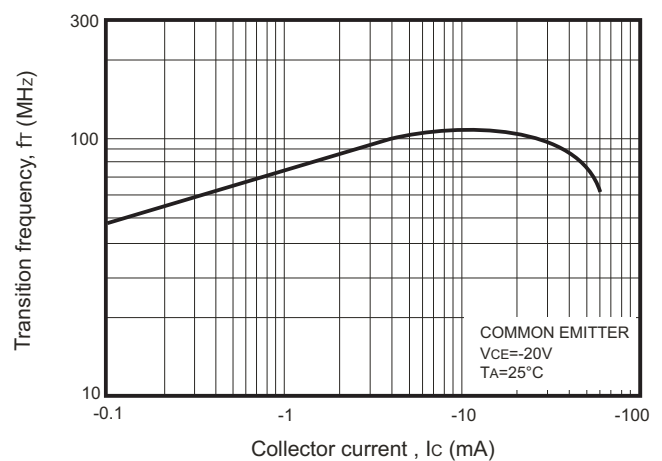
Fig.6 - f_T - I_c
