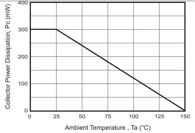
Fig. 8- P_c - T_a
