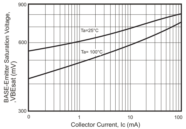
Fig.4- V_{BEsat} - I_c
