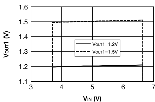
Output voltage - Input voltage (1)
