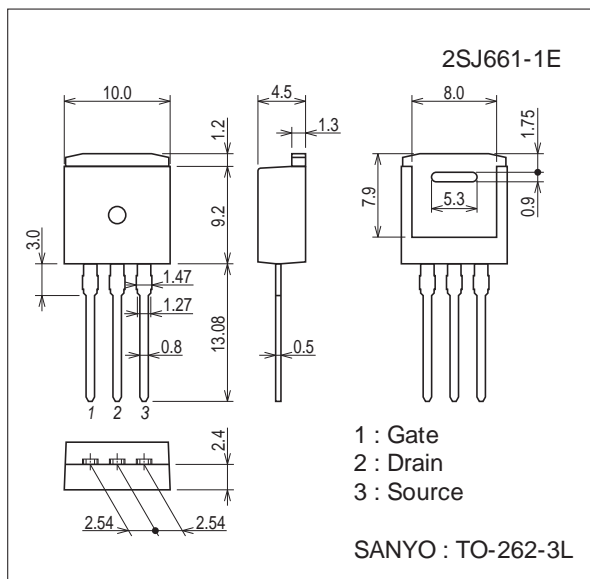
Package Dimensions unit : mm (typ) 7537-001
