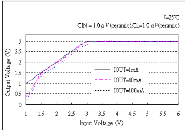
ML6206S302
