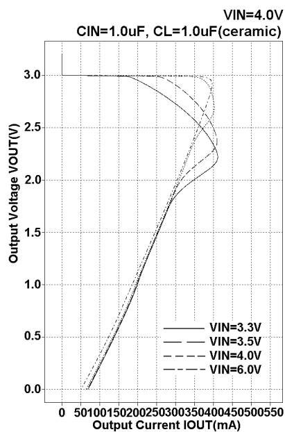
ML6206S302
