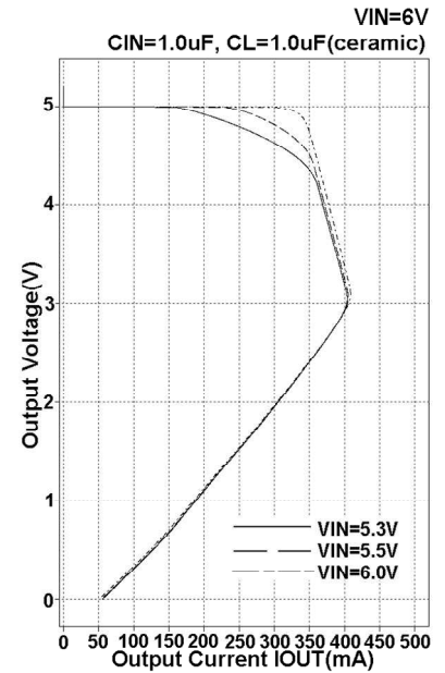
ML6206S502
