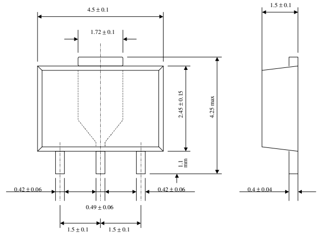
SOT-89 :
