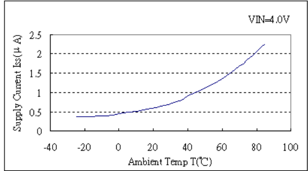
ML6206S302
