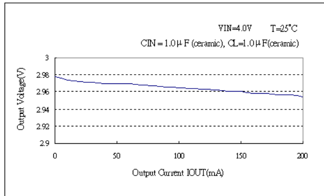
ML6206S302
