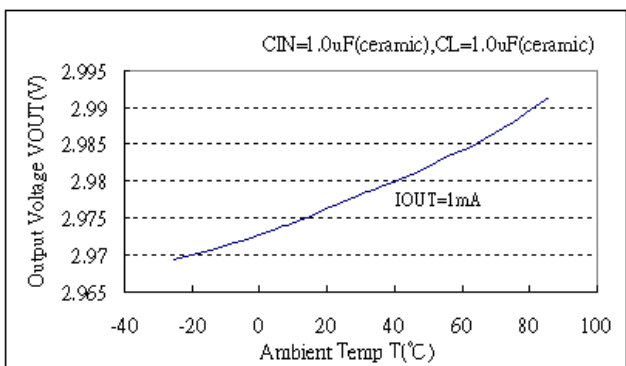
ML6206S302
