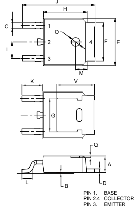
DIMENSIONS
