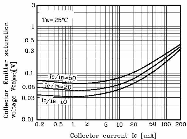
Fig. 5 V_{CE(sat)} - I_C
