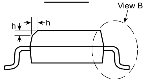
View A-A
