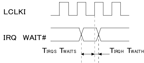
図27. ローカル入力信号(IRQ、WAIT#)のセットアップ、ホールド時間
