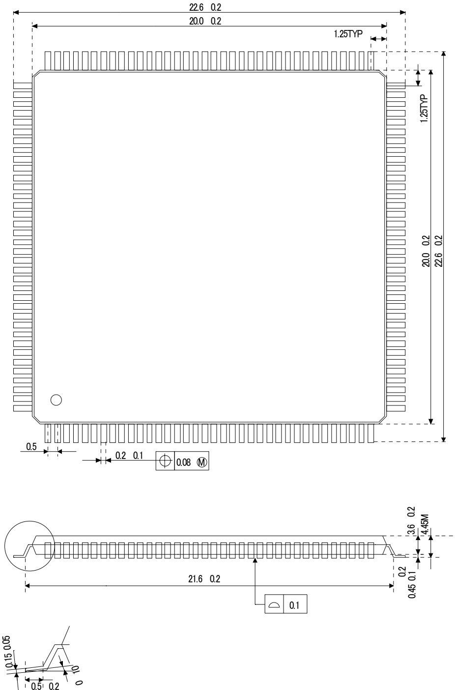
図32. 外形寸法図
