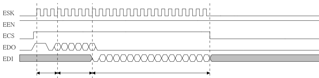
図17. EEPROMタイミングチャート
