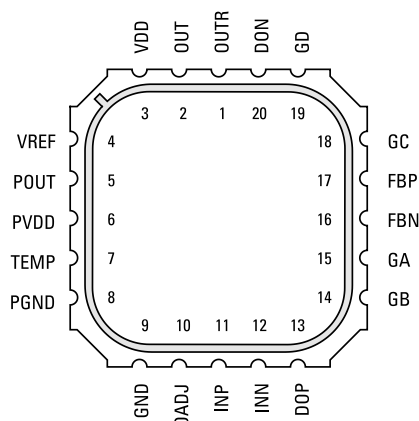
20L CQFN Pinout
