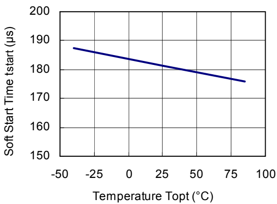
RP503x15xA
