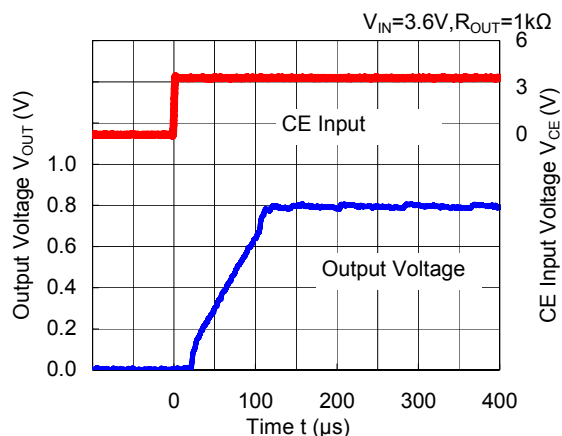
RP502x081B/083B
