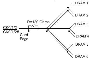
*Clock Net Wiring
