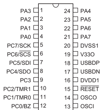
HT82A851R - 24 SSOP-A
