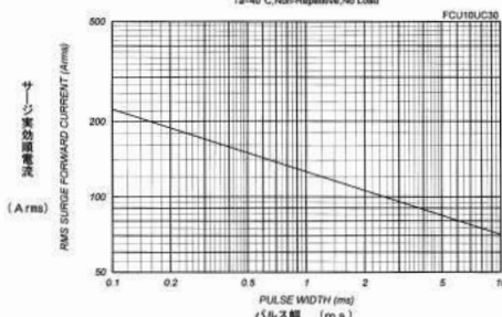
FIG.5 サージ実効順電流定格 RMS SURGE CURRENT RATINGS
