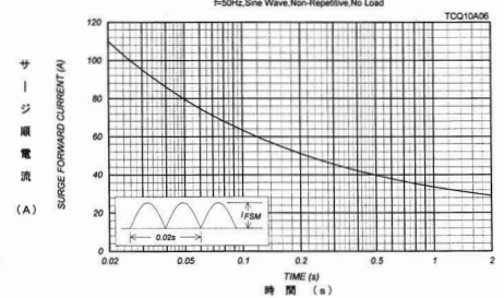
サージ順電流定格 SURGE CURRENT RATINGS
